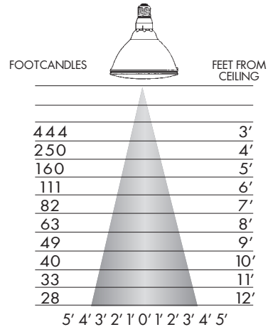
90 WATT PAR 38 FLOOD BEAM ANGLE = 30°
