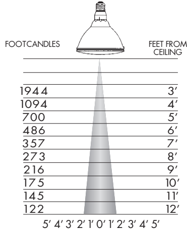
75 WATT PAR 38 SPOT BEAM ANGLE = 10°
