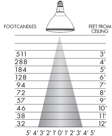
120 WATT PAR 38 FLOOD BEAM ANGLE = 30°
