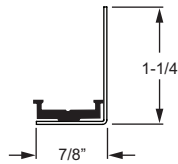
90° Reflector
