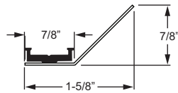
45° Reflector
